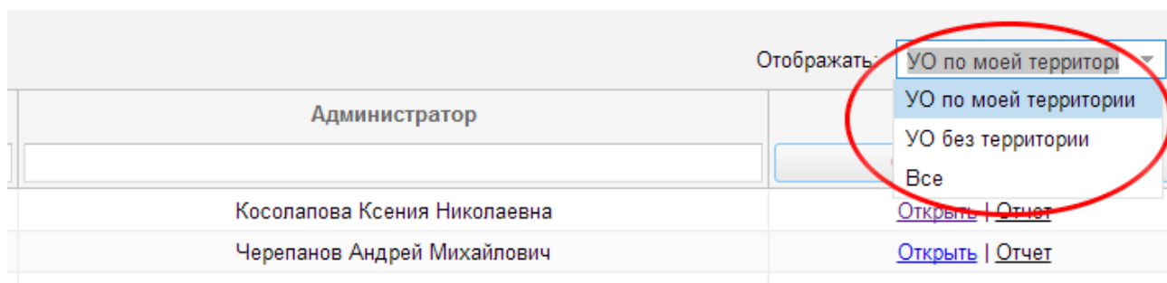
Рисунок 7 – Фильтр списка
