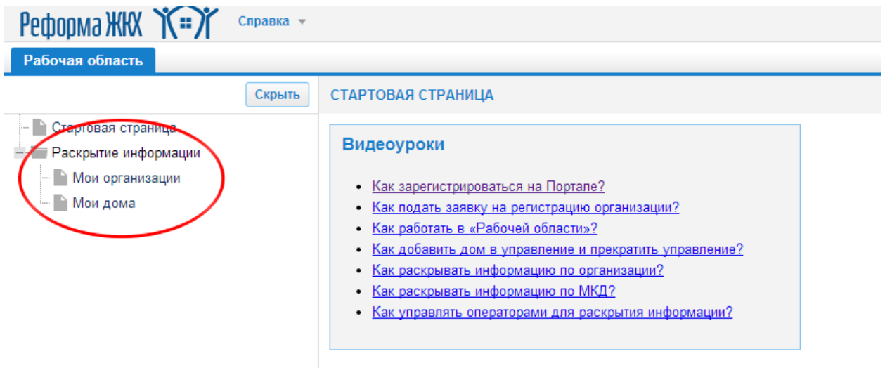
Рисунок 5 – Рабочая область
